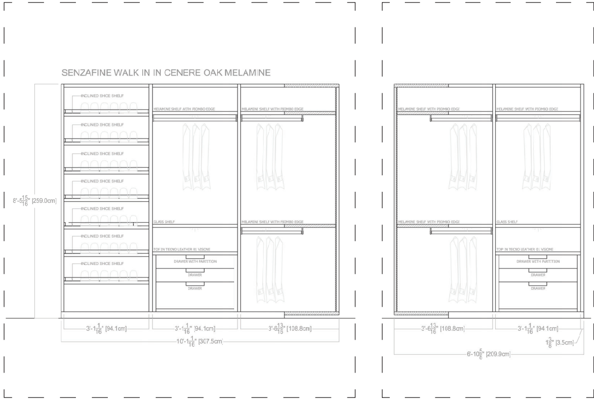
SENZAFINE - ELEVATION A & B
